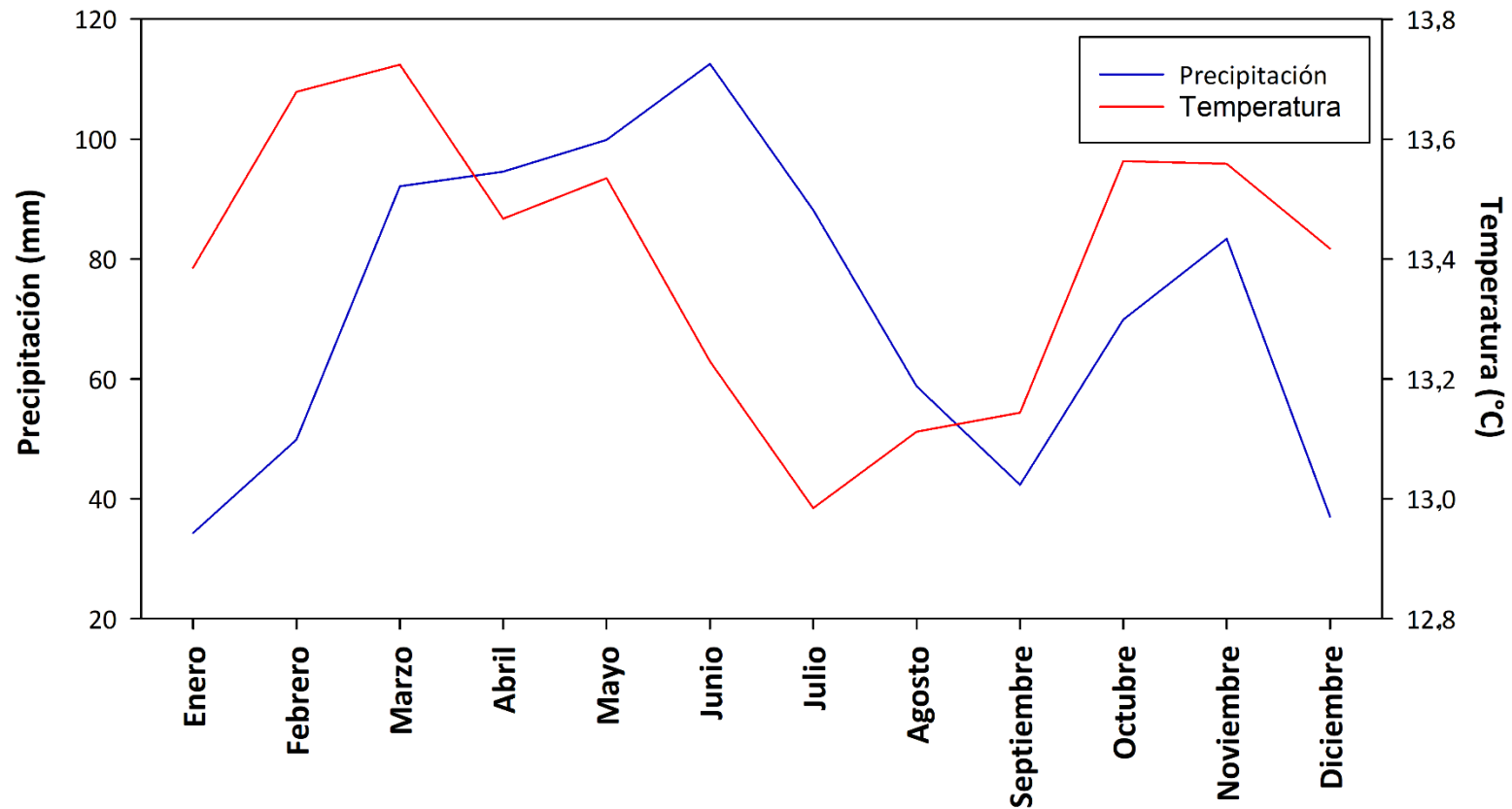
Anexo 2. Variación de la precipitación y temperatura en Guasca, Cundinamarca, a partir de un promedio multianual (2015-2025). Estación meteorológica “Guasca” (4°52'40,63” N, 73°51'52,03” O).
